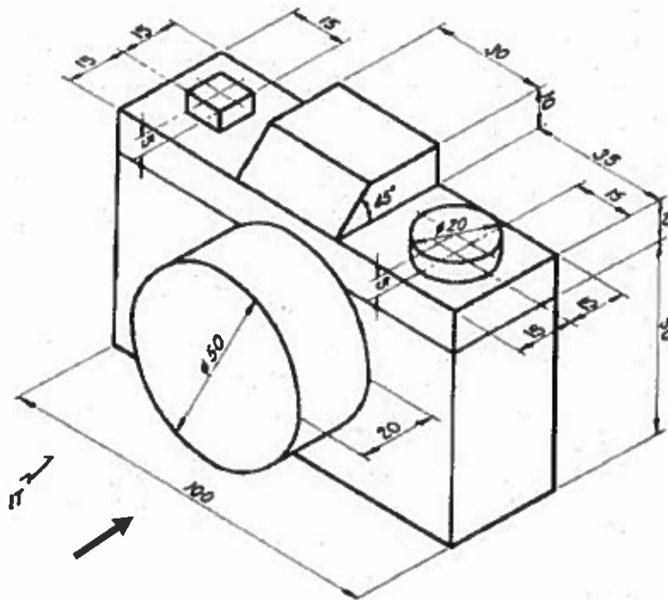
Fig.1 - Desenho da estrutura de uma máquina fotográfica em perspectiva isométrica e cotada em centímetros.
